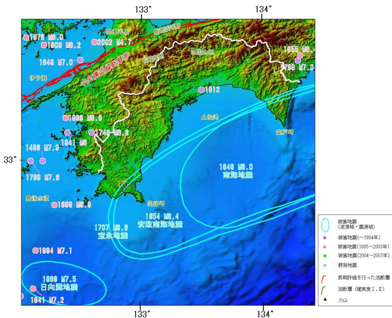
高知県とその周辺で発生した主な被害地震と活断層位置
