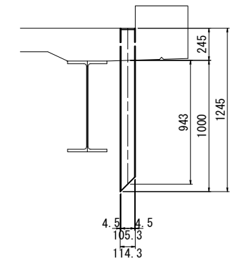
排水施設詳細図 S=1:20
