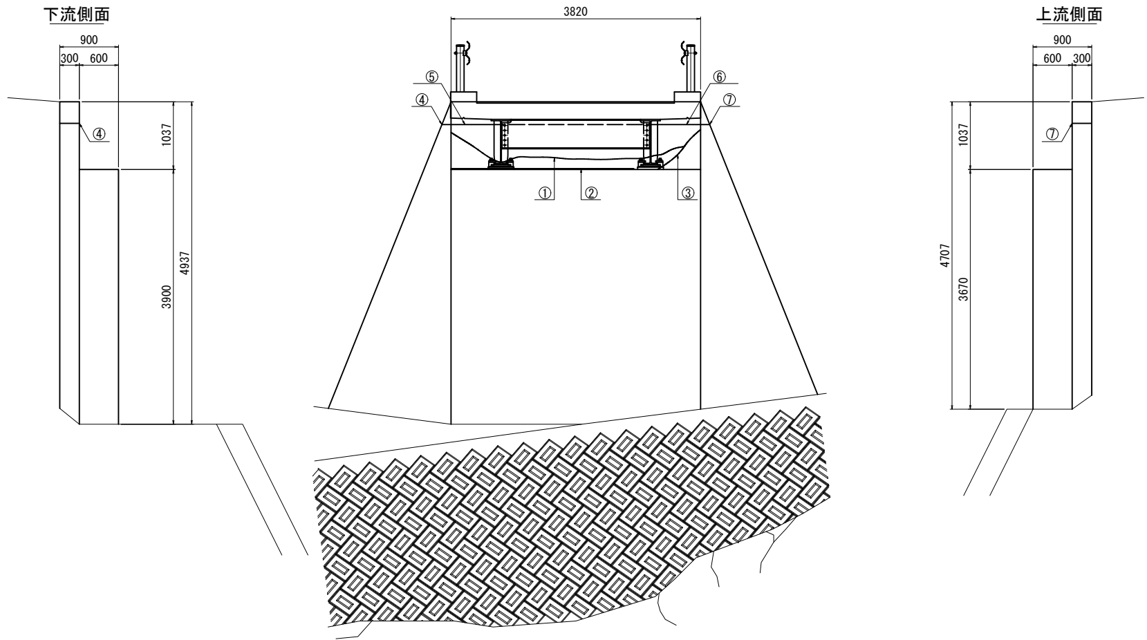
A2橋台 S=1:40
