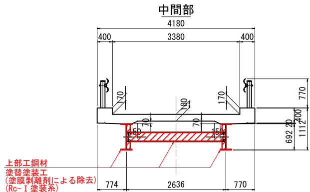
断面図 S=1:50
