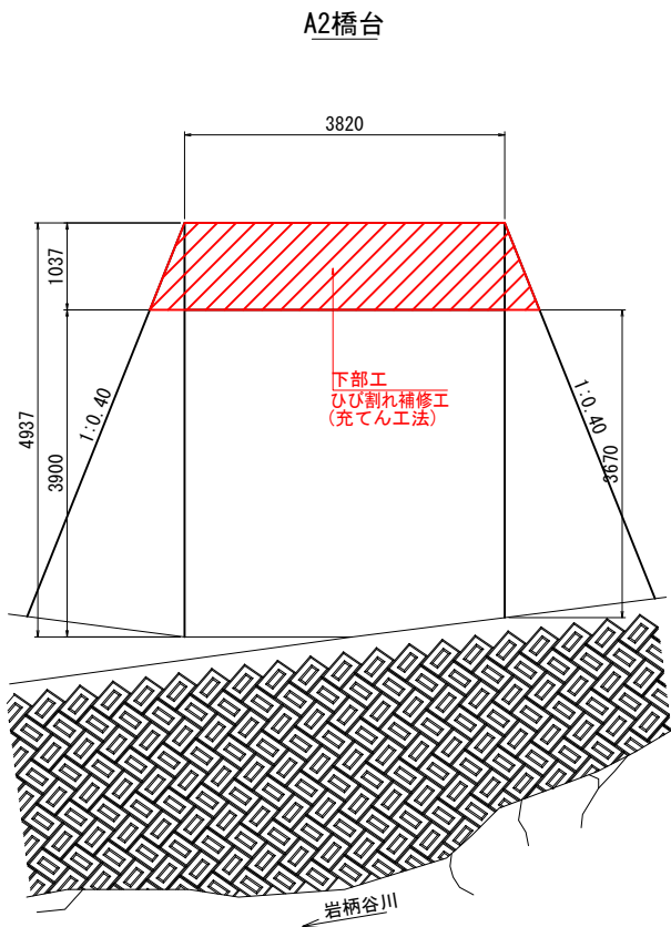
下部工正面図 S=1:50
