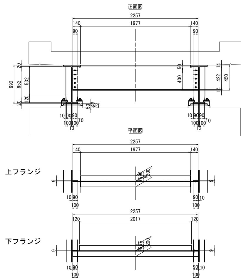
終点側端横桁詳細図 S=1:20
