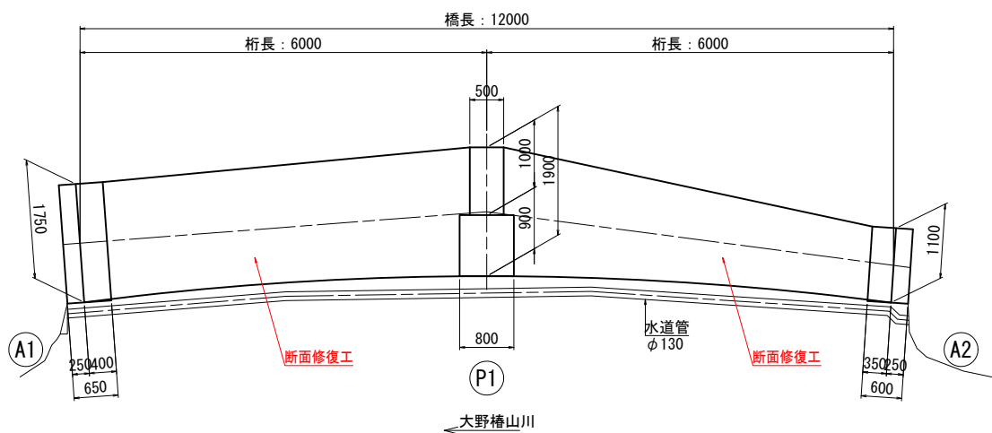
桁下面図 S=1:50
