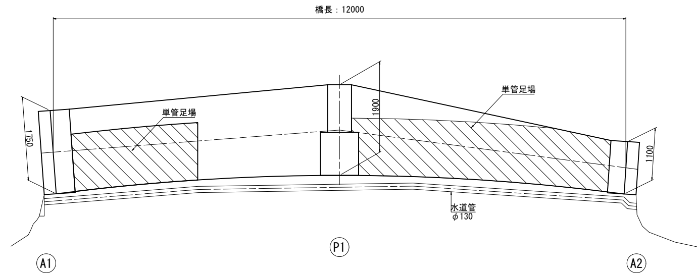
平面図 S=1:40
