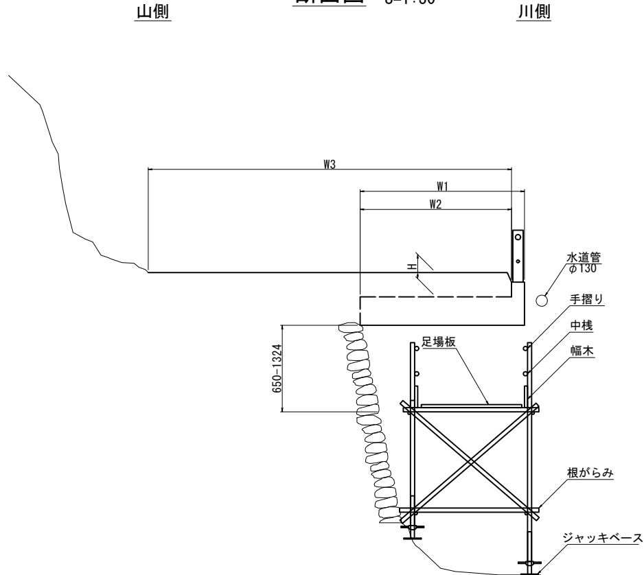
断面図 S=1:30
