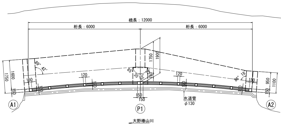
平面図 S=1:50
