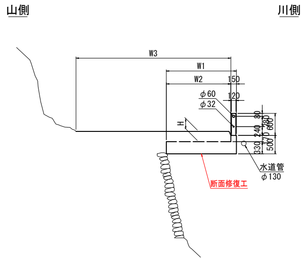
断面図 S=1:50
