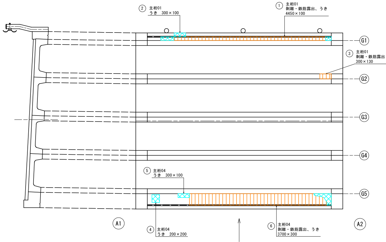
断面修復工詳細図 (左官工法)
