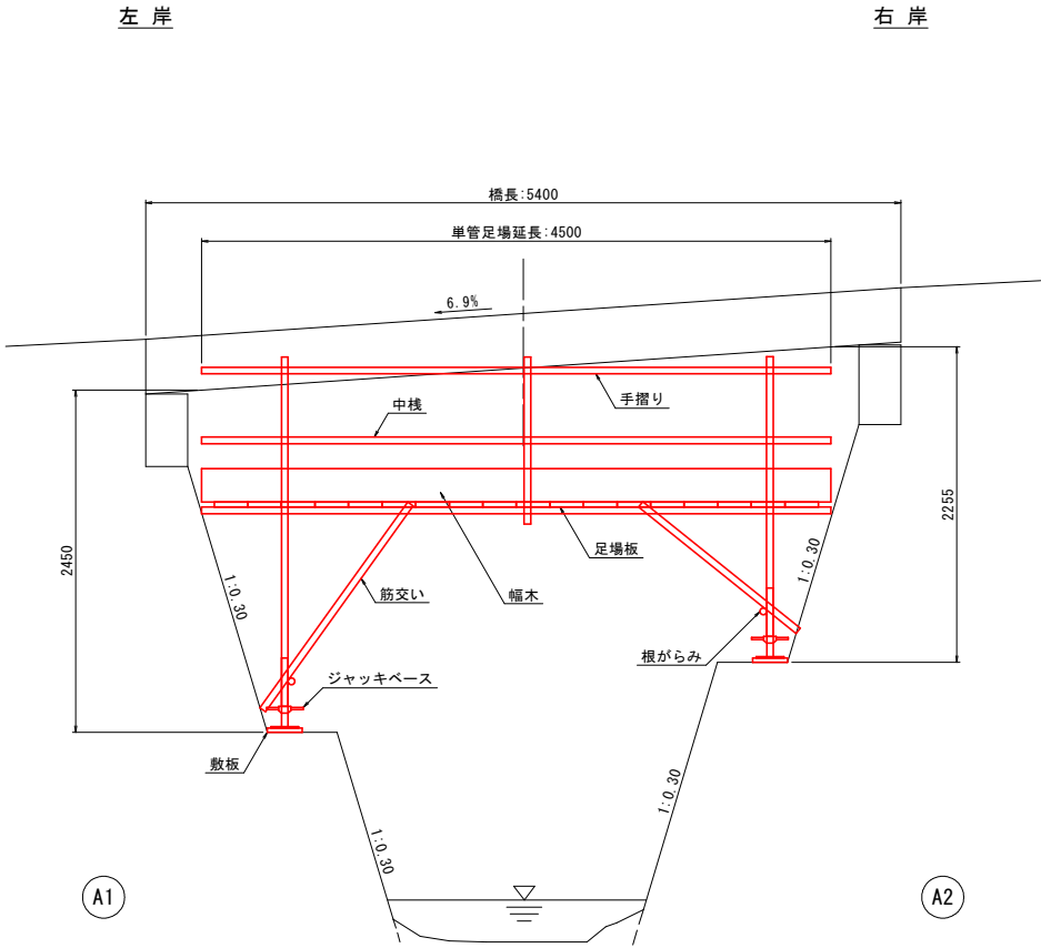
側面図 S=1:30
