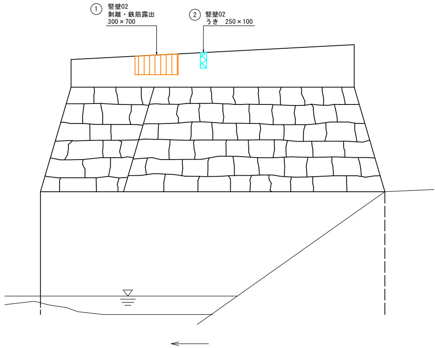
A2橋台 S=1:30
