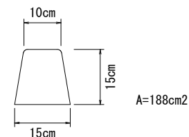
アスカープ詳細図 S=1:10
