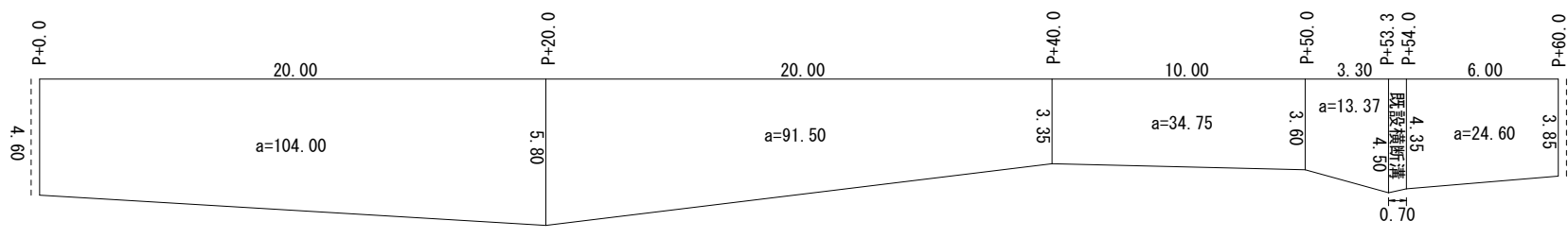
アスカープ詳細図 S=1:10
