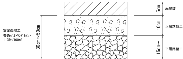
舗装構成図
