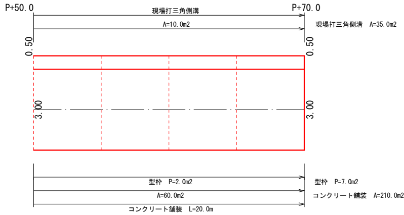
標準断面図
