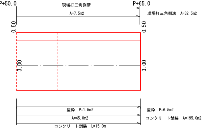
標準断面図
